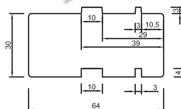
WKŁADKA TERMICZNA POD PRÓG ALUMINIOWY
